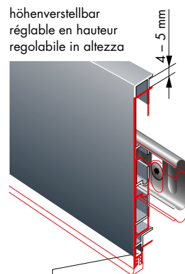
höhenverstellbar réglable en hauteur regolabile in altezza
