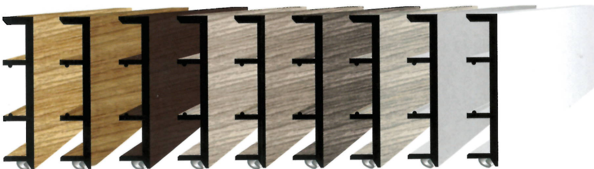
Die beiden kubischen Formate von 40 x 12 und 60 x 12 mm sind mit einer Gummilippe ausgestattet und verhindern das Eindringen von Staub und Feuchtigkeit.
