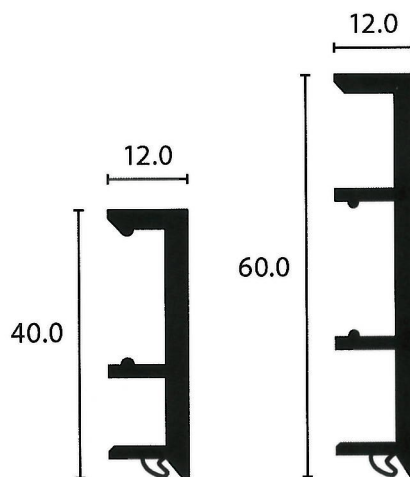
Die beiden kubischen Formate von 40 x 12 und 60 x 12 mm sind mit einer Gummilippe ausgestattet und verhindern das Eindringen von Staub und Feuchtigkeit.
